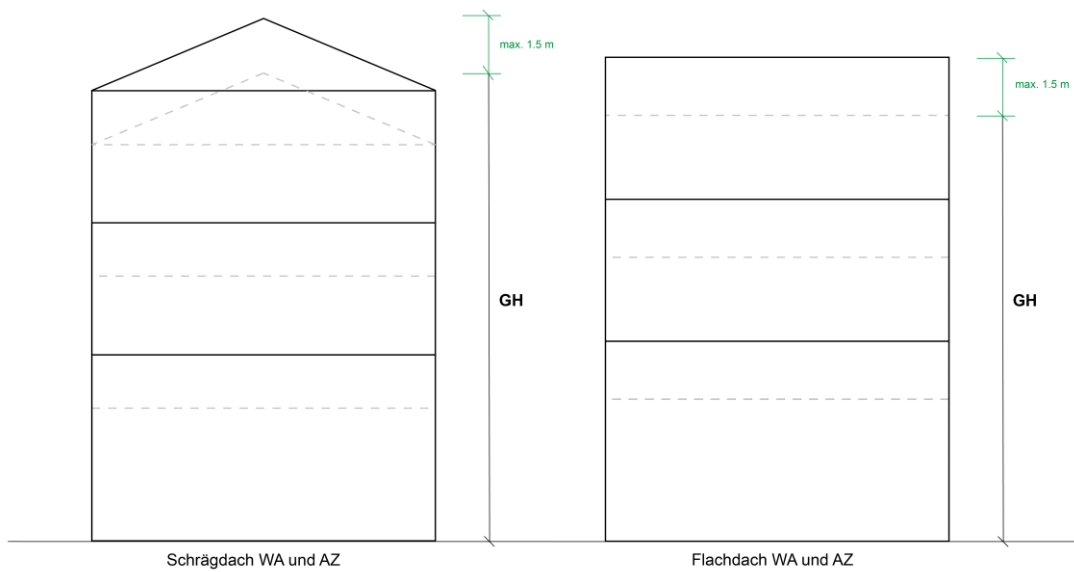
Abb. 1: Art. 61 Abs. 1 Gesamt- und Fassadenhöhe
