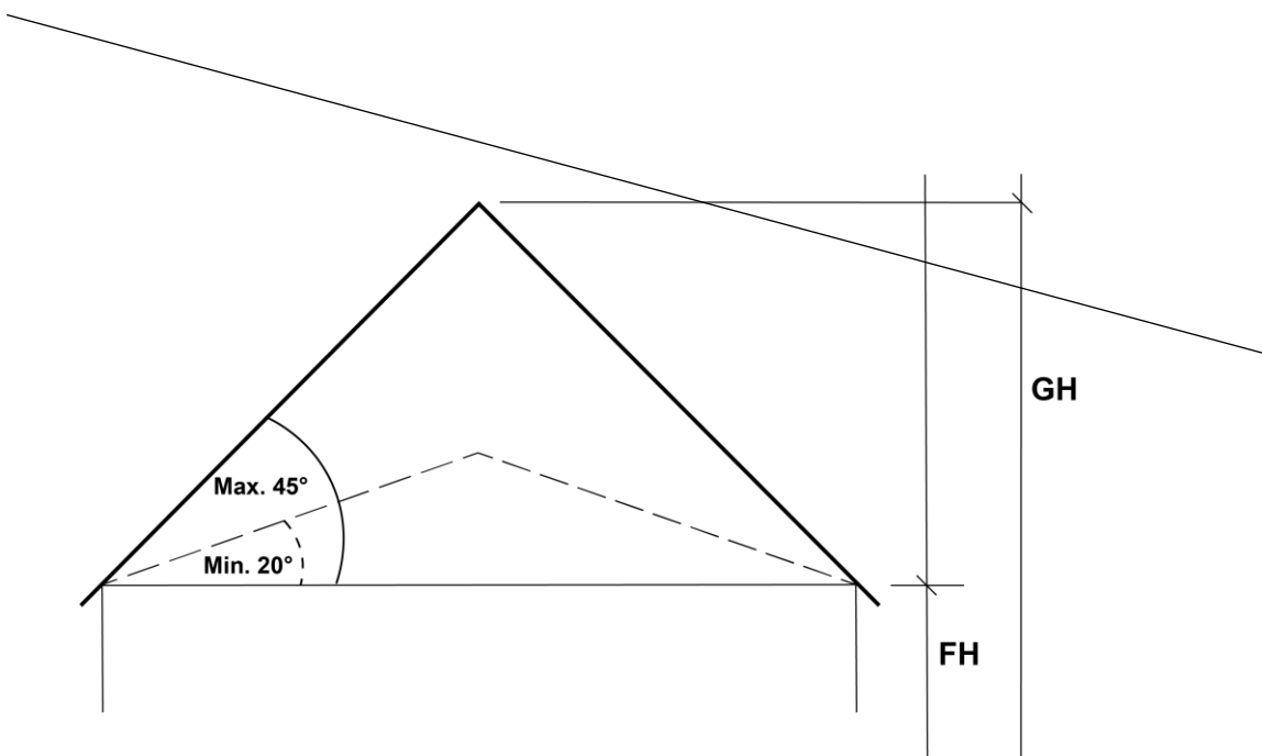
Abb. 3: Art. 63 Abs. 1 Schrägdachbauten
