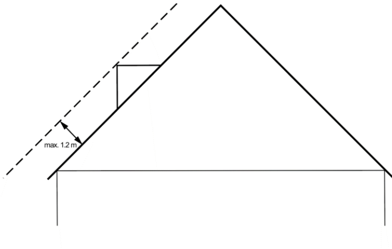
Abb. 4: Art. 63 Abs. 4 Schrägdachbauten
