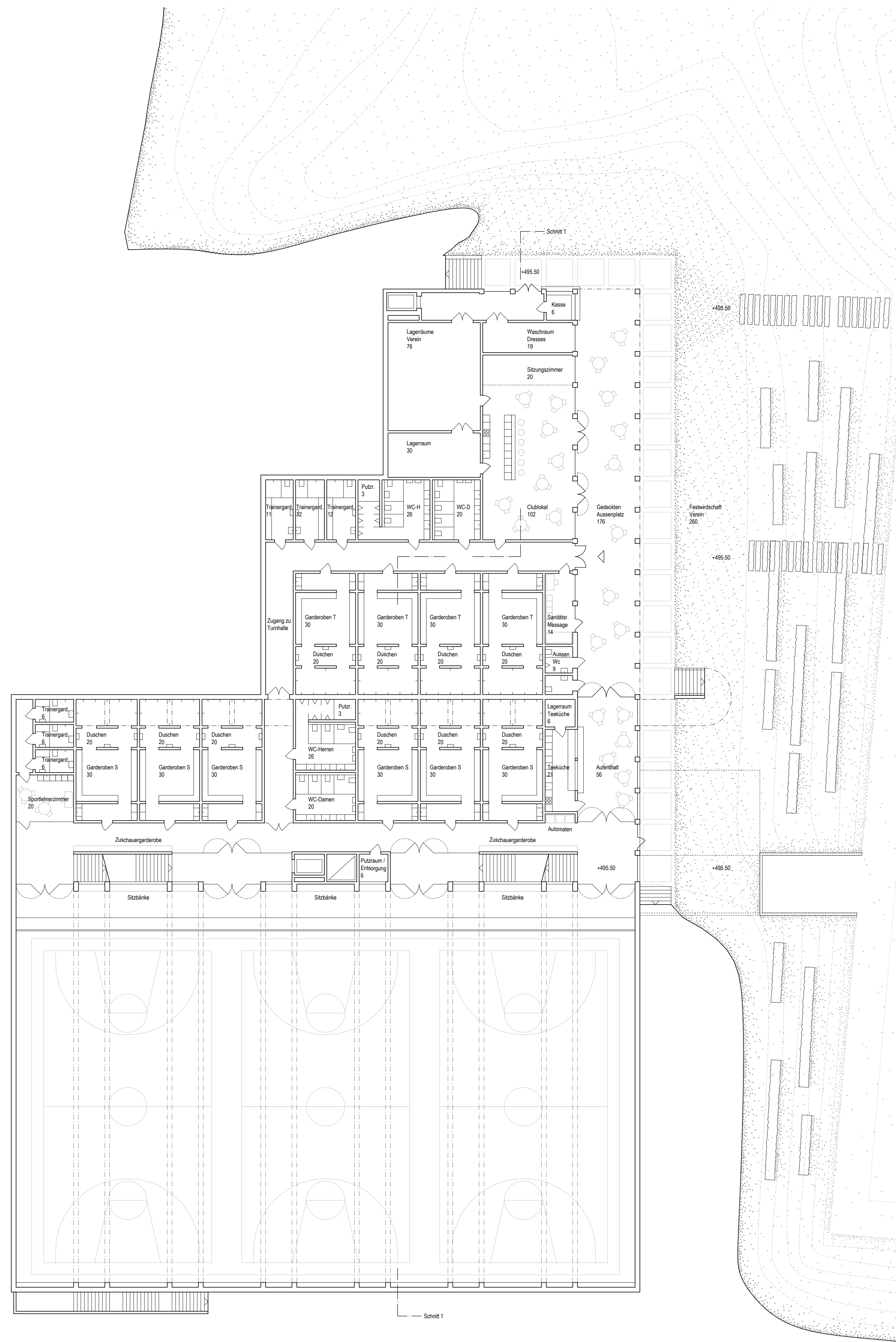
2. Untergeschoss Turnhalle 1:200
