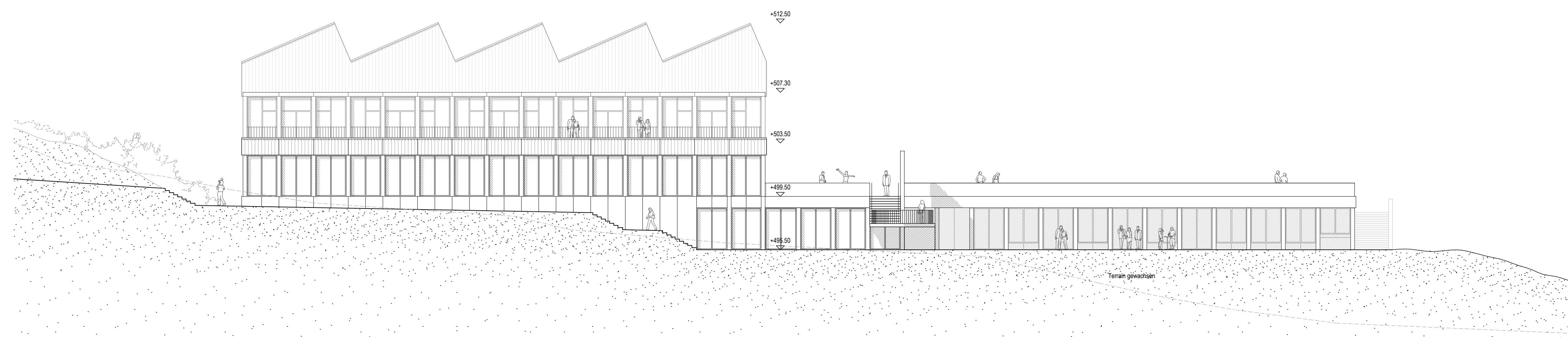
Ansicht Ost Turnhalle 1:200
