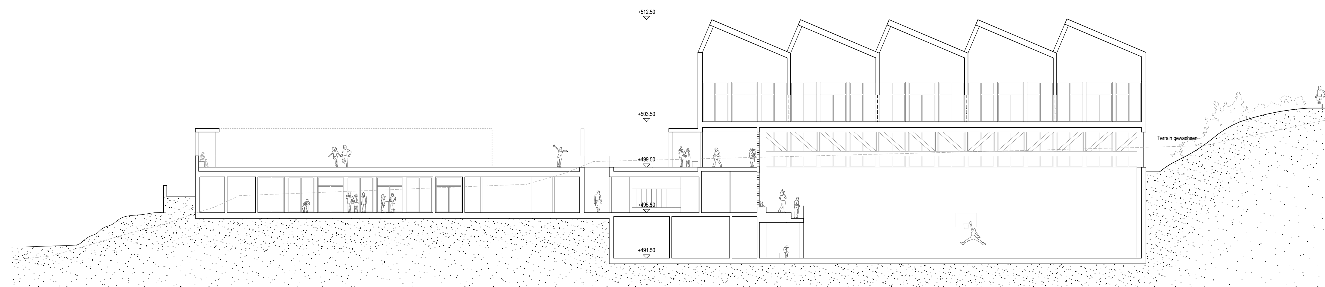
Schnitt 1 Turnhalle 1:200
