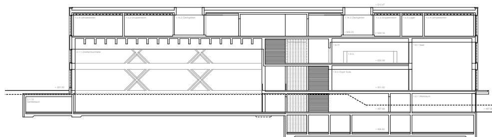
Schnitt B-B
