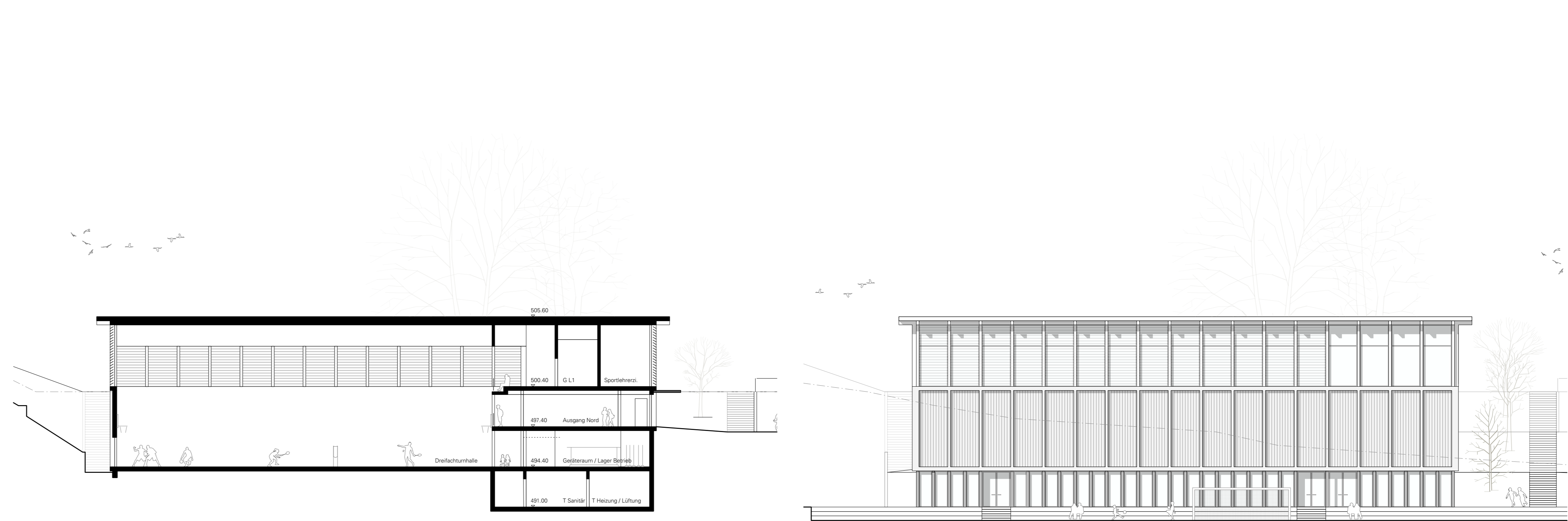
Schnitt 06
