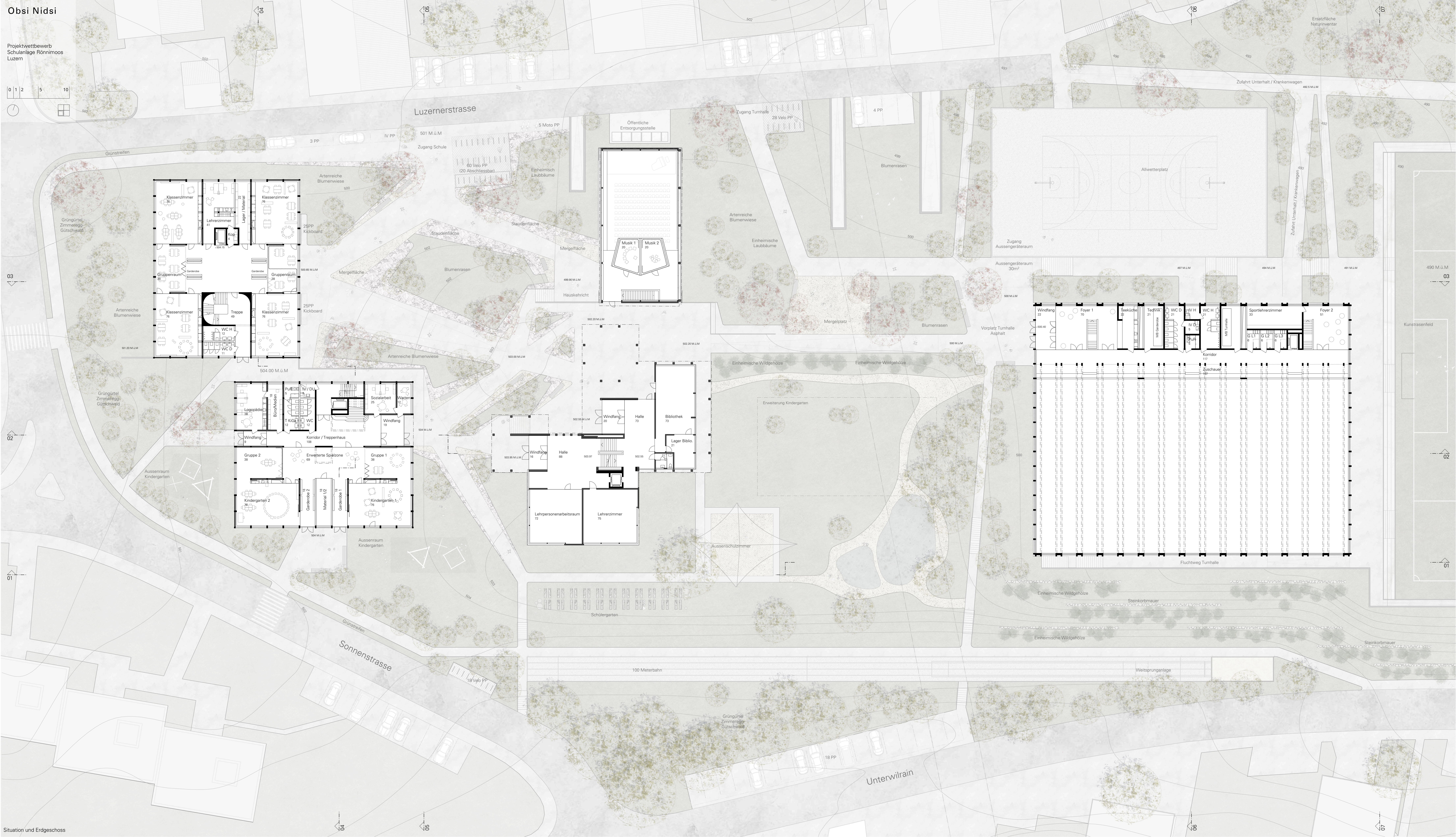
Situation und Edgeschoss
