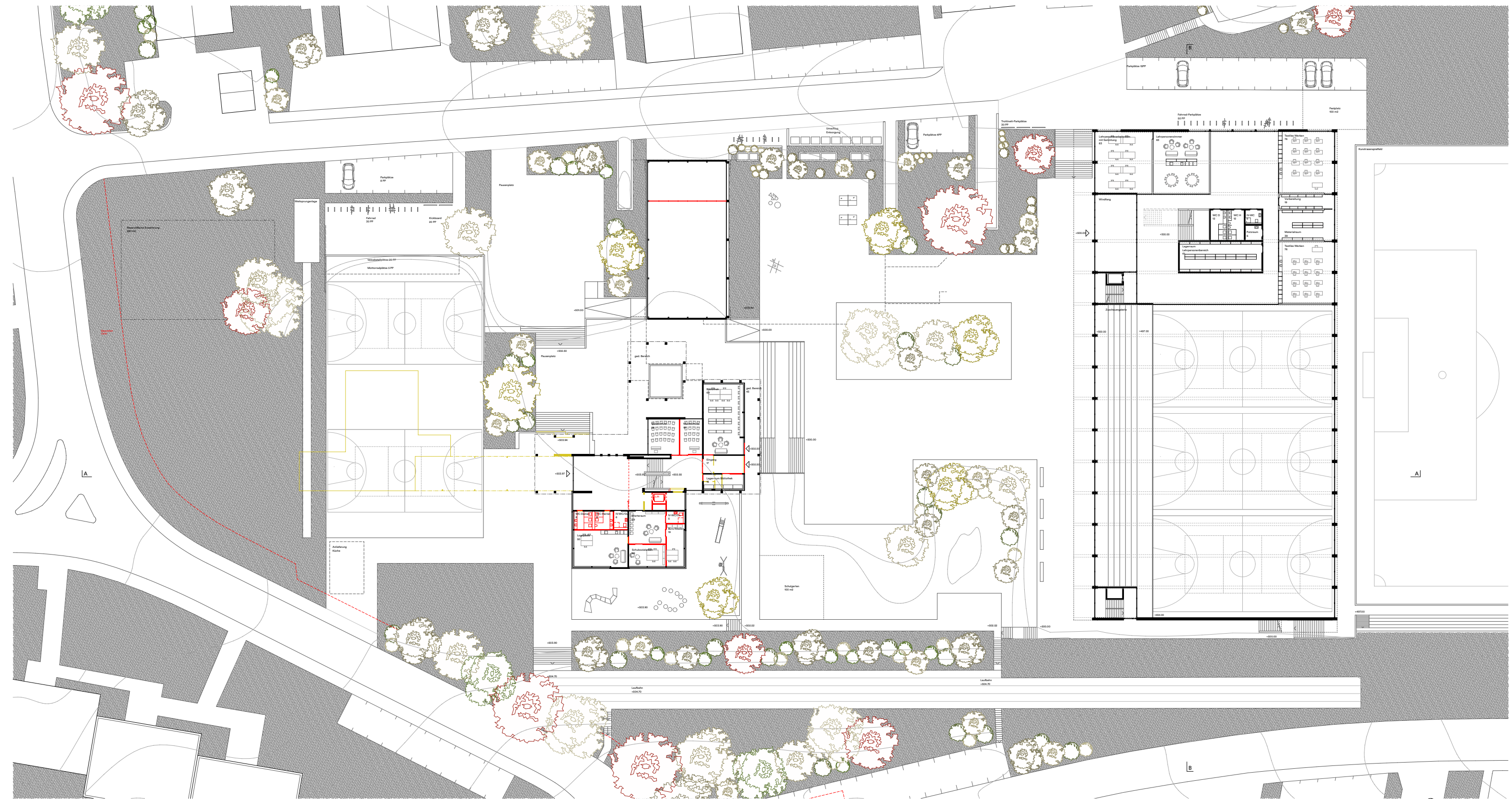
Erdgeschoss 1:200
