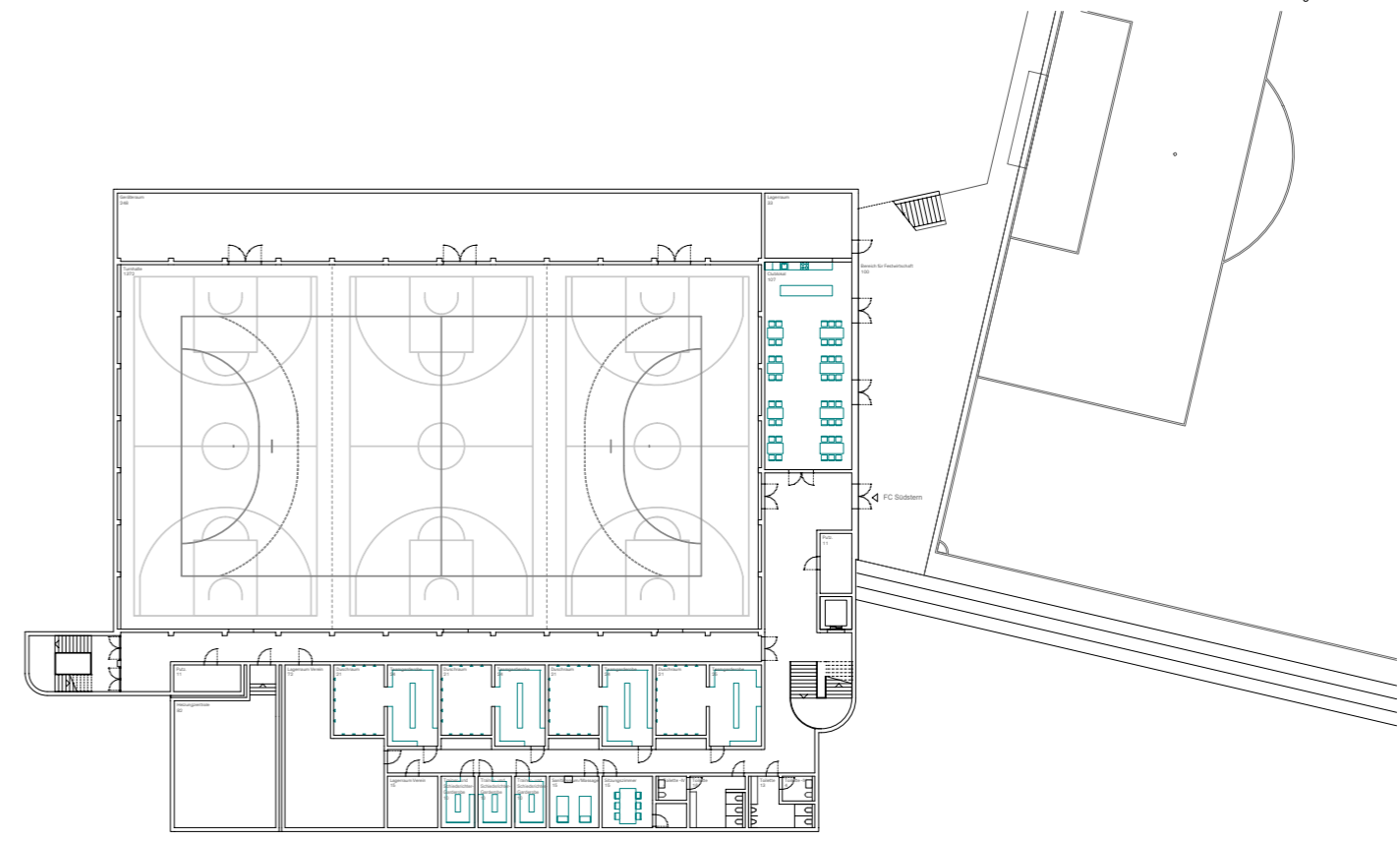
Turnhalle 2. Untergeschoss 1.200
