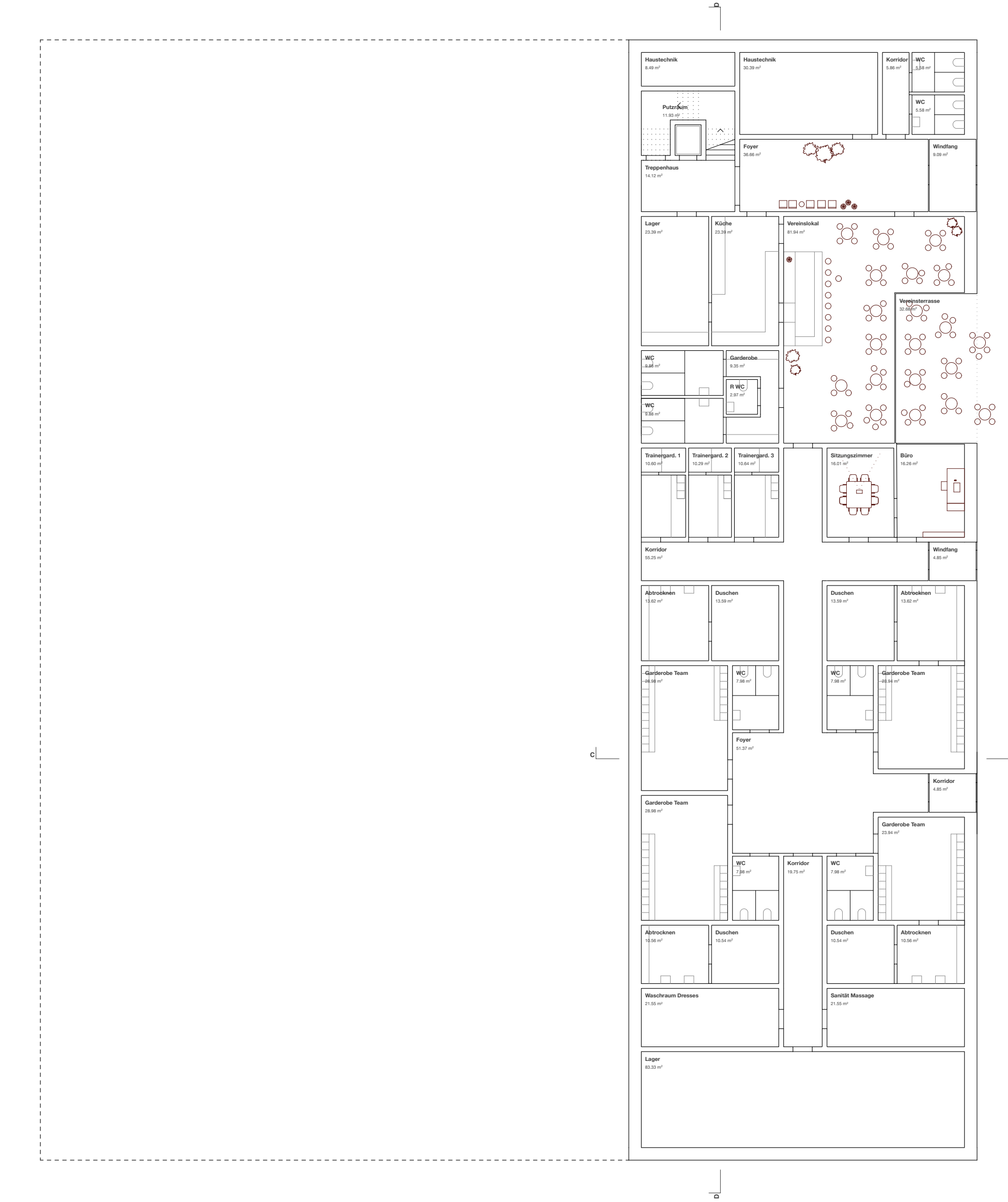
Grundriss Sporthalle 2. Untergeschoss, M 1:200
