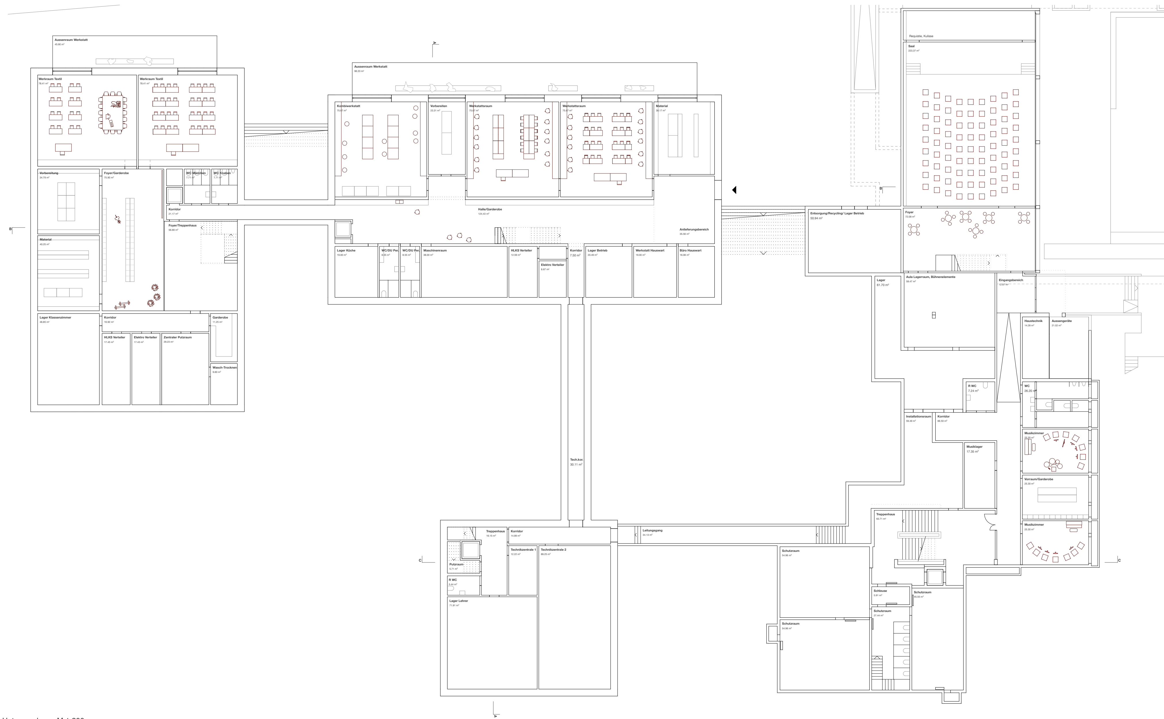
Grundriss 1. Untergeschoss, M 1:200
