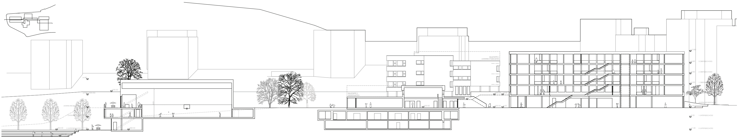
SCHNITT AA
