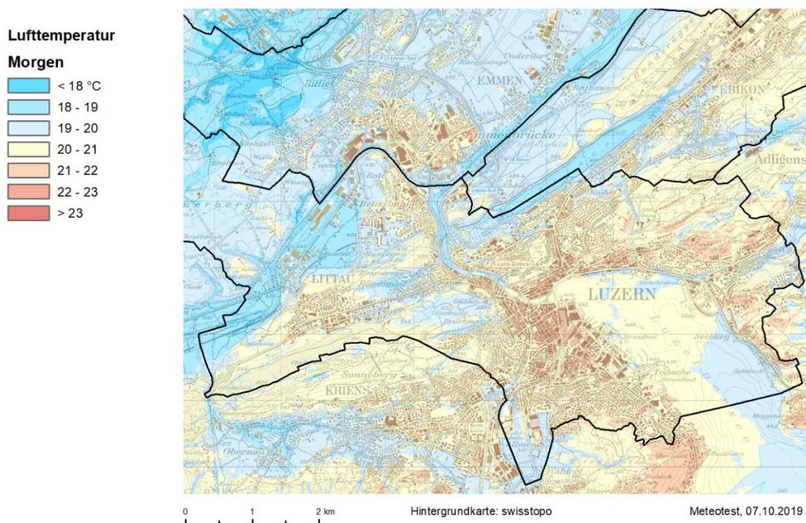
Abb. 4: Lufttemperatur frühmorgens (vor Sonnenaufgang) 2 m über Grund. Mittel über fünf Hitzetage (24 Std.). Quelle: Klimaanalyse Stadt Luzern 2019
