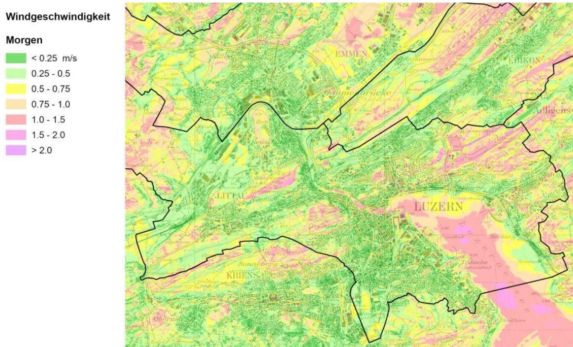
Abb. 6: Windgeschwindigkeit frühmorgens (vor Sonnenaufgang) 2 m über Grund. Mittel über fünf Hitzetage (24 Std.). Quelle: Klimaanalyse Stadt Luzern 2019
