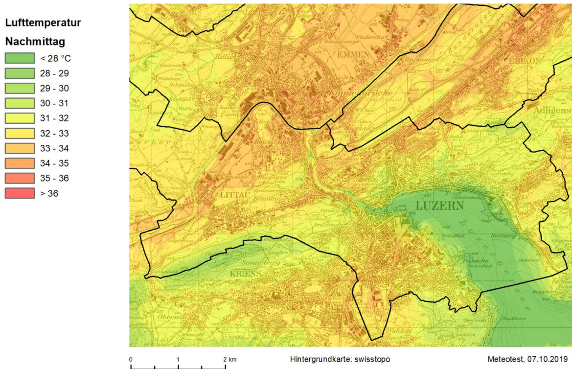
Abb. 5: Lufttemperatur zum heissesten Zeitpunkt des Tages (zwischen 16 und 17 Uhr MESZ) 2 m über Grund. Mittel über fünf Hitzetage (24 Std.). Quelle: Klimaanalyse Stadt Luzern 2019
