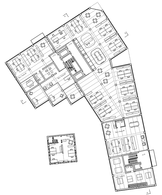
1. OBERGESCHOSS 1:200
