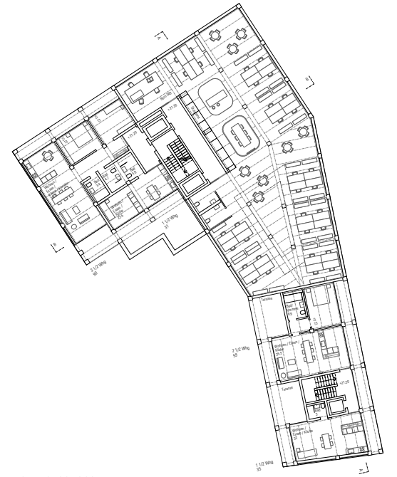
7. OBERGESCHOSS 1:200
