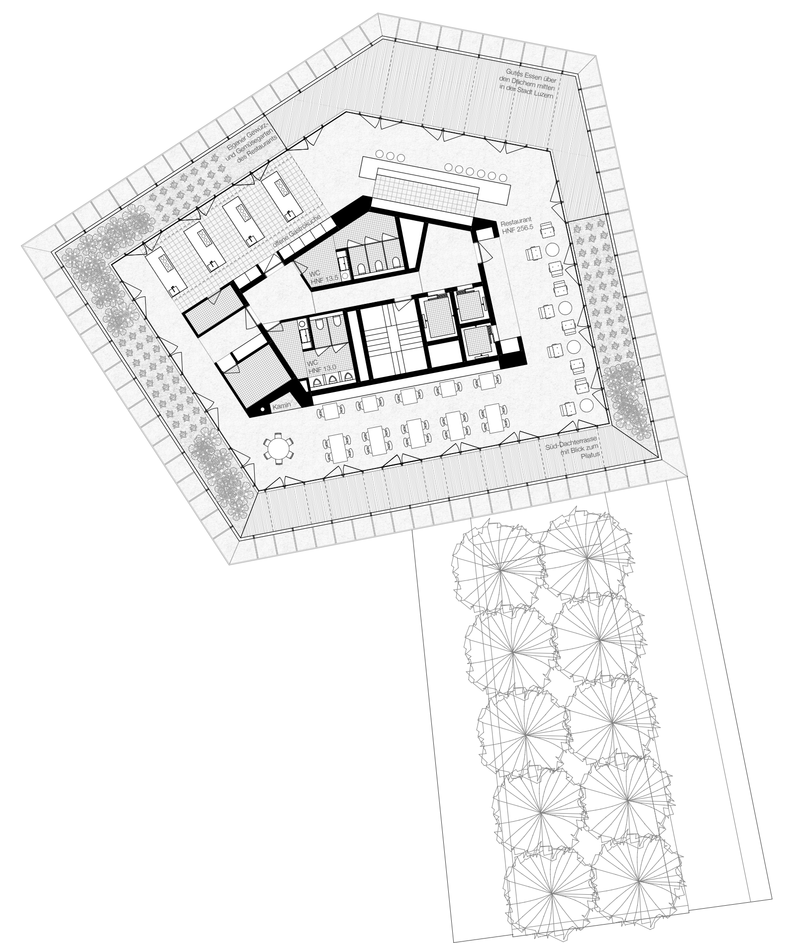
Dachgeschoss 1:200
