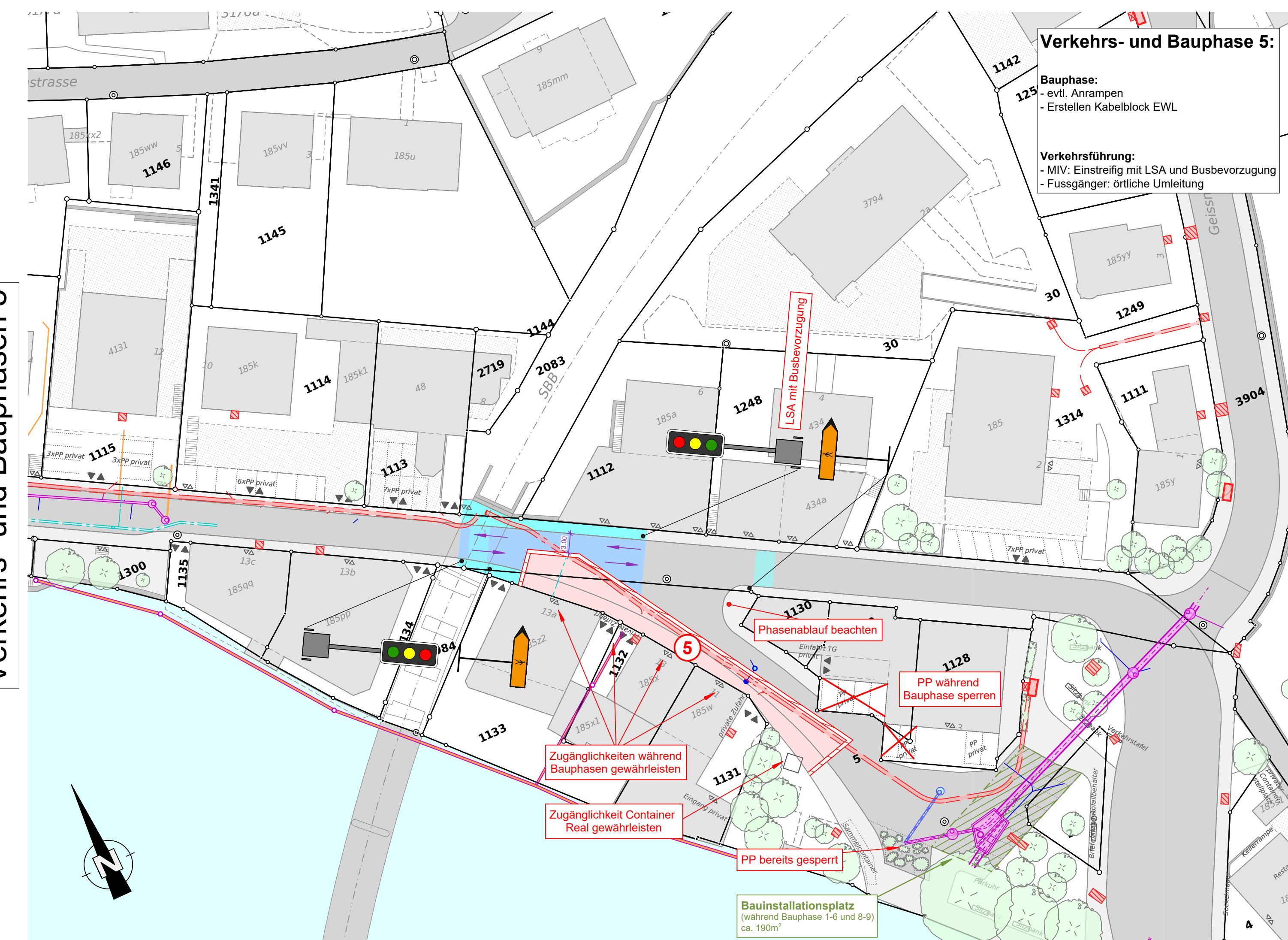
Verkehrs- und Bauphasen 5
