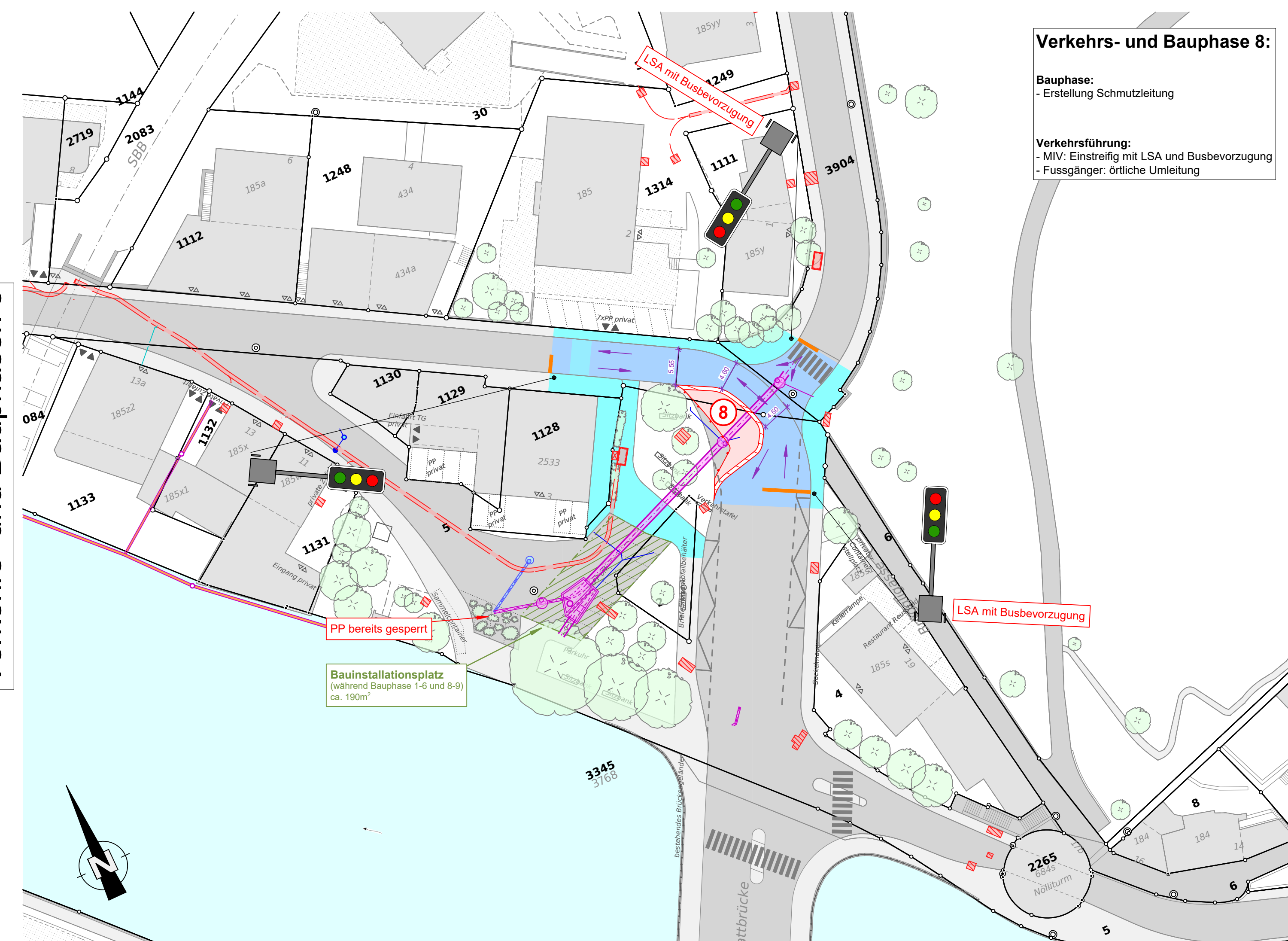
Verkehrs- und Bauphasen 8
