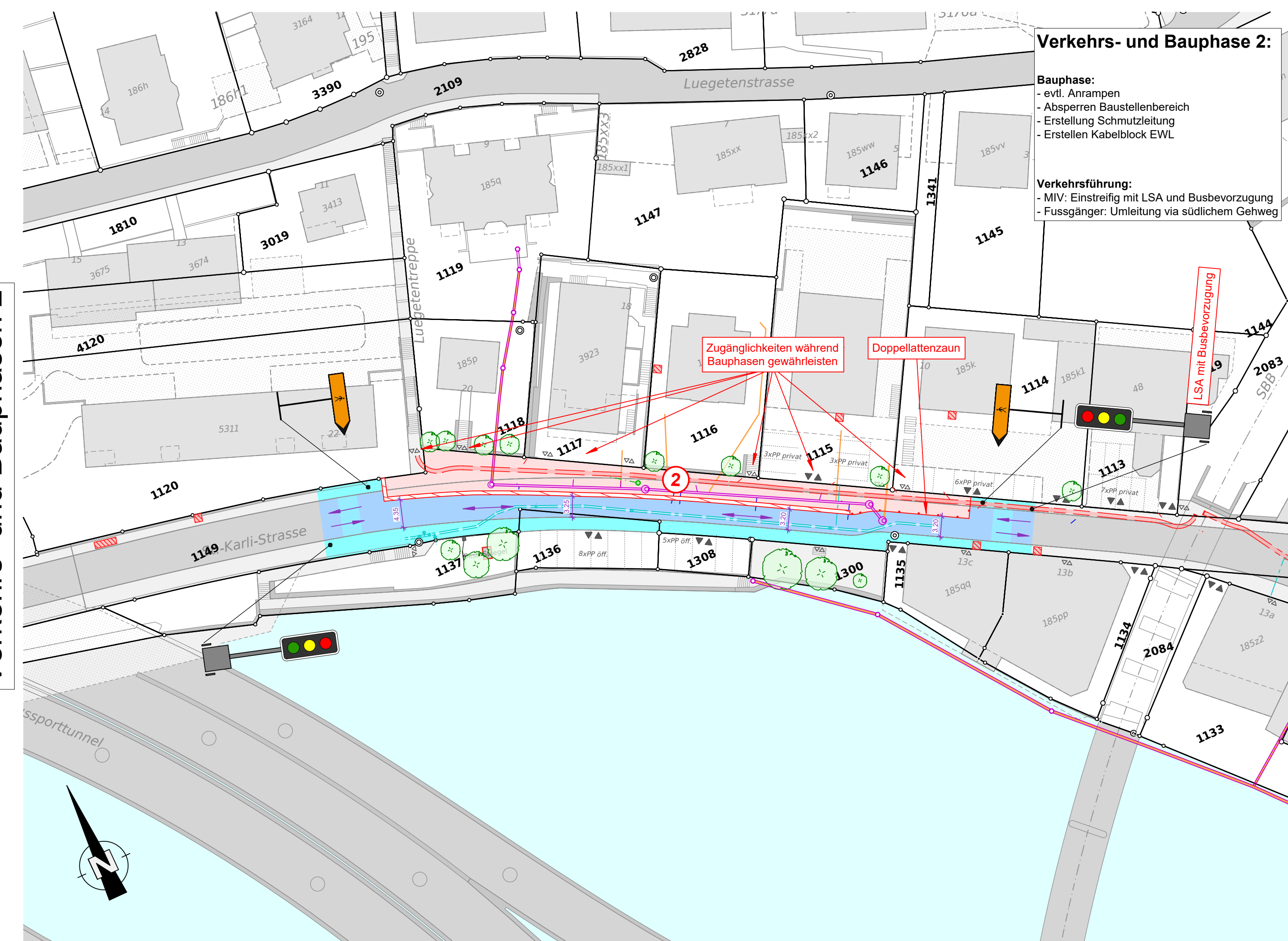
Verkehrs- und Bauphasen 2
