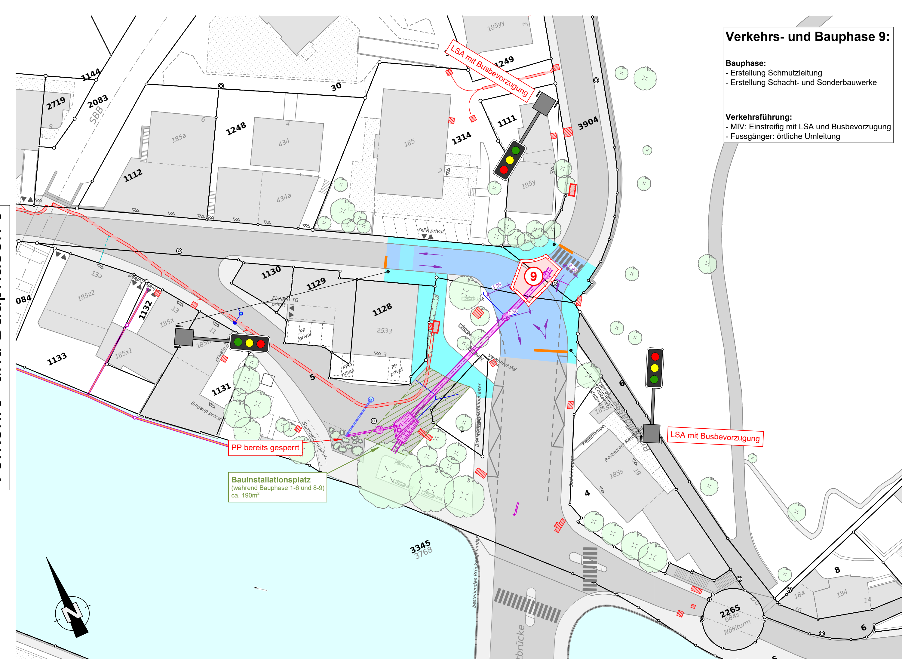
Verkehrs- und Bauphasen 9
