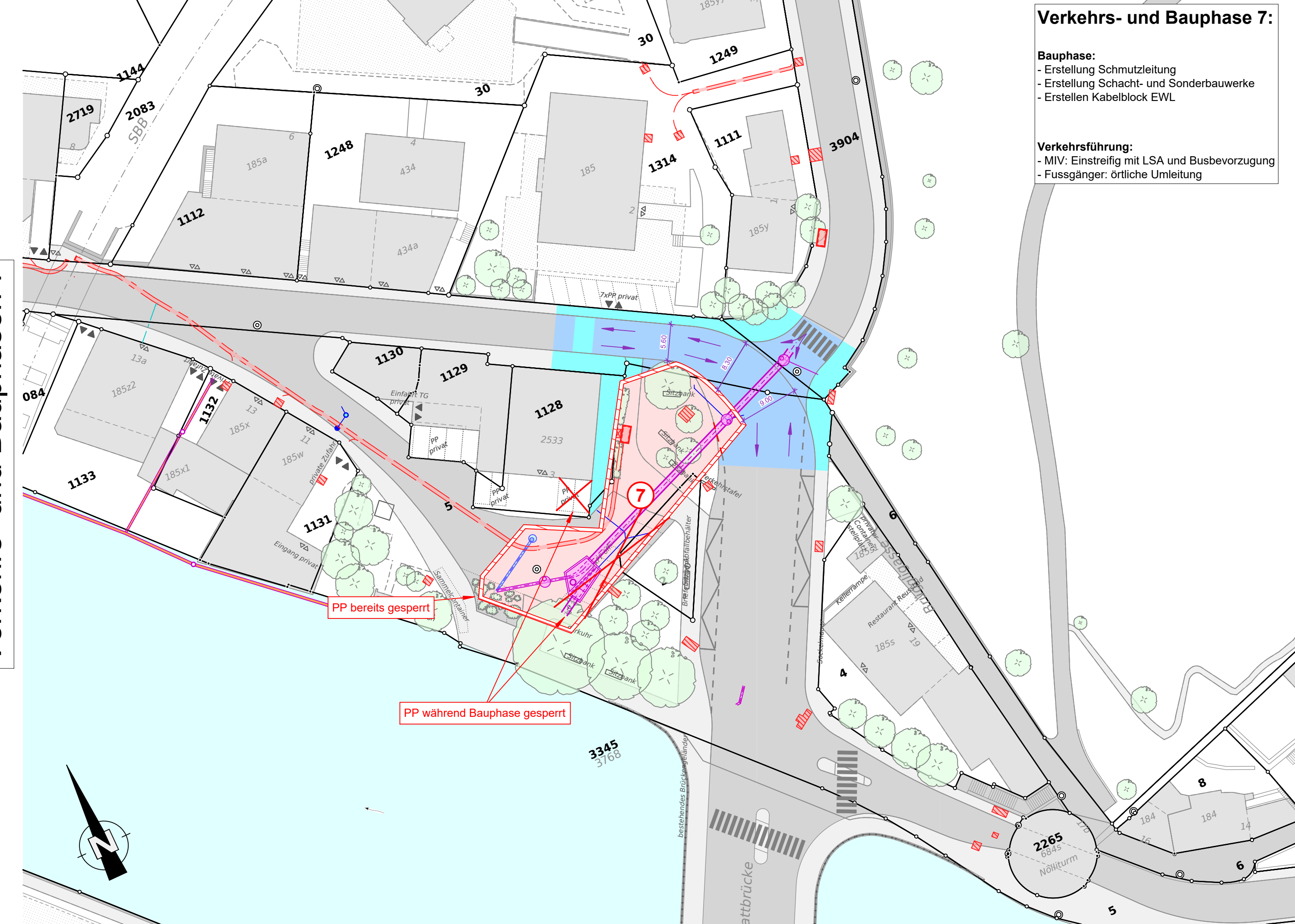
Verkehrs- und Bauphasen 7
