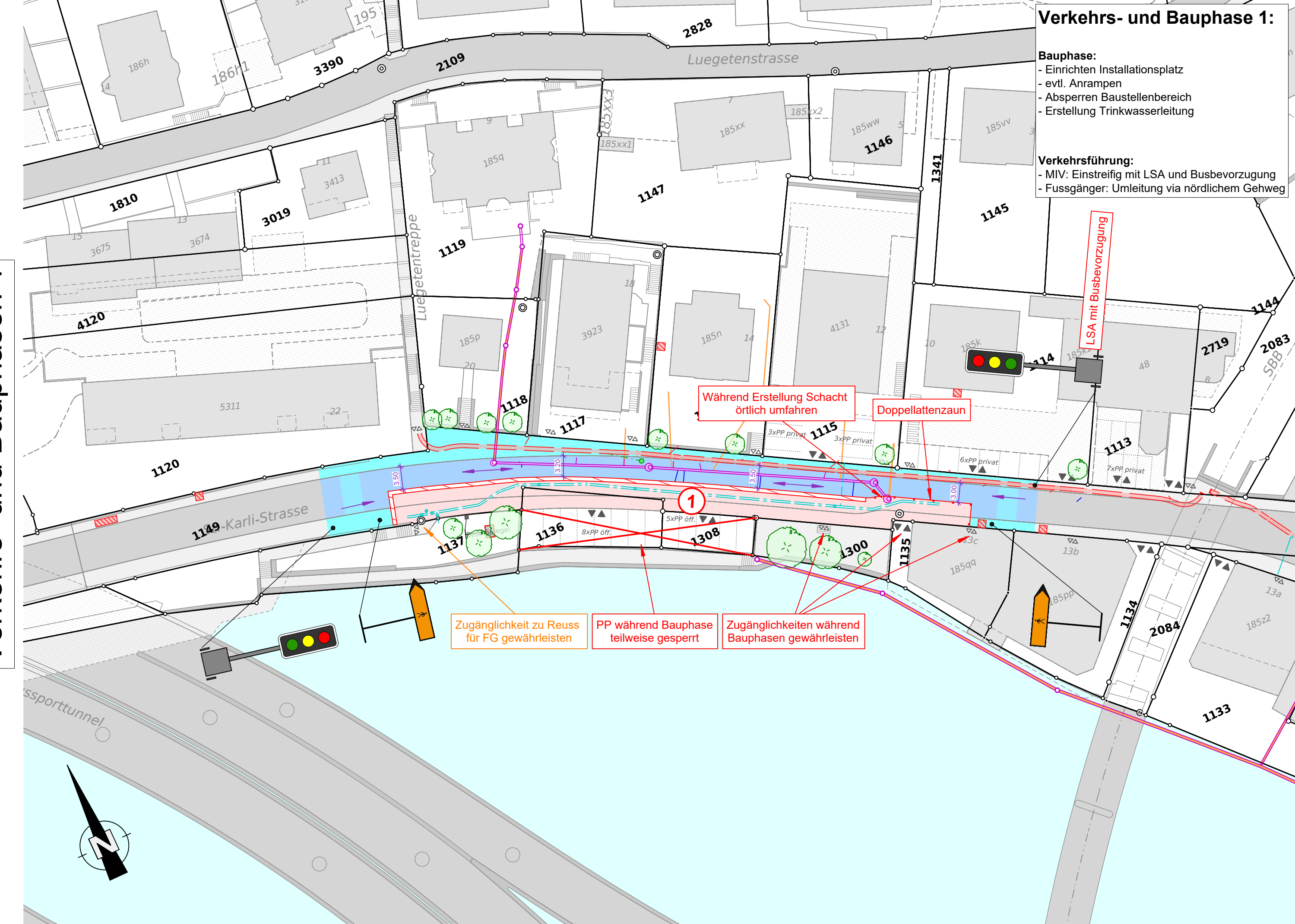
Verkehrs- und Bauphasen 1
