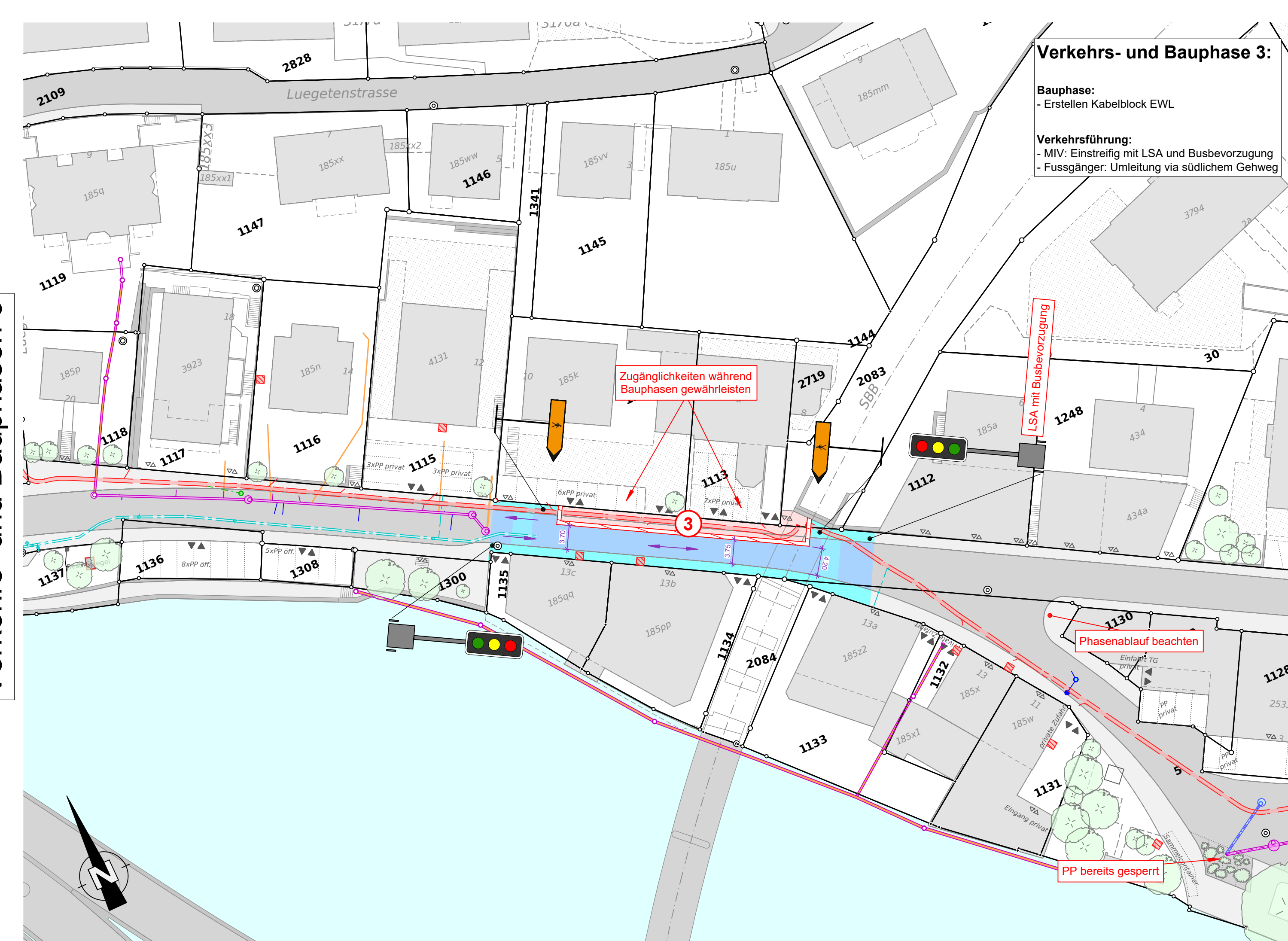
Verkehrs- und Bauphasen 3
