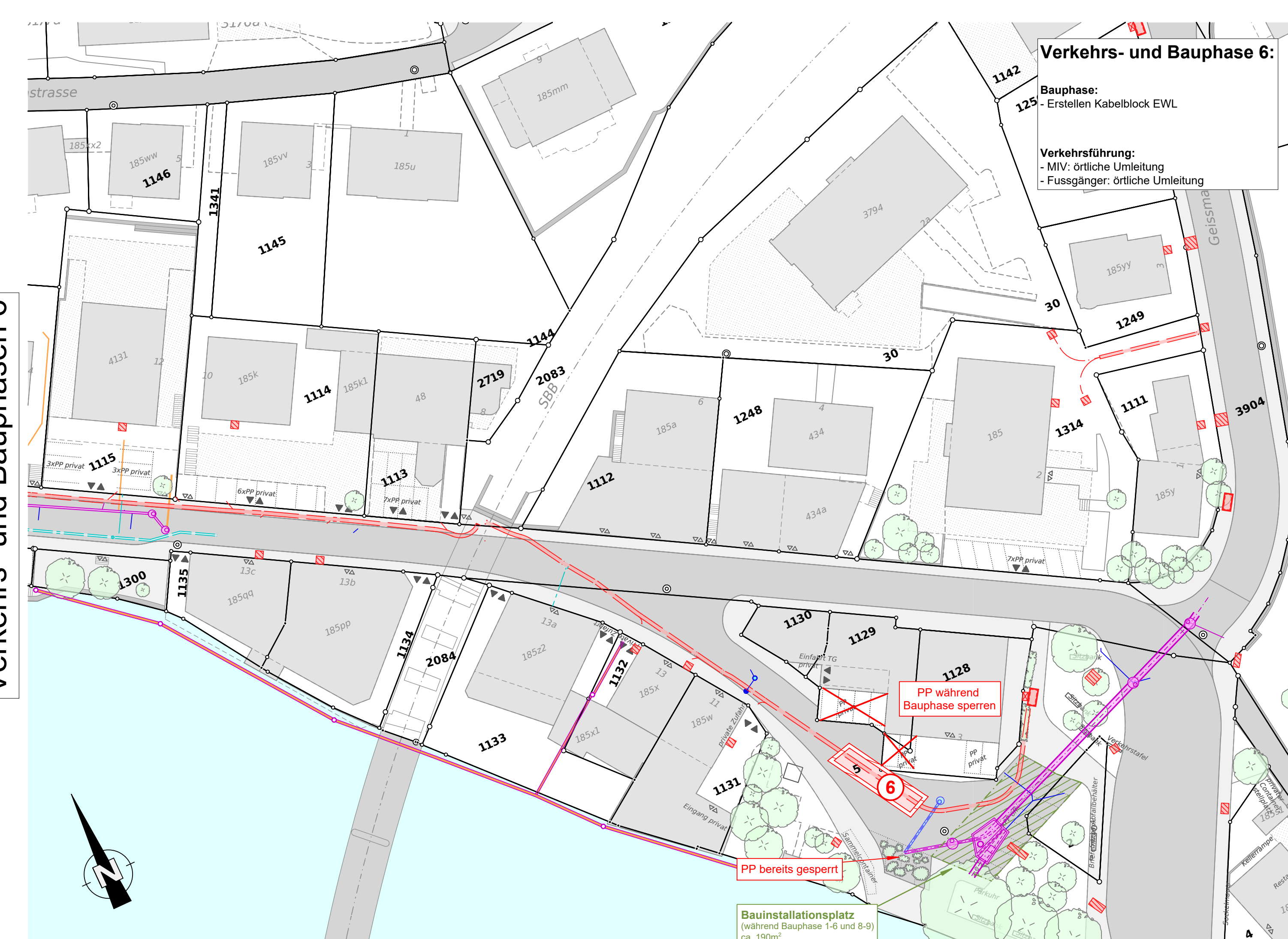
Verkehrs- und Bauphasen 6
