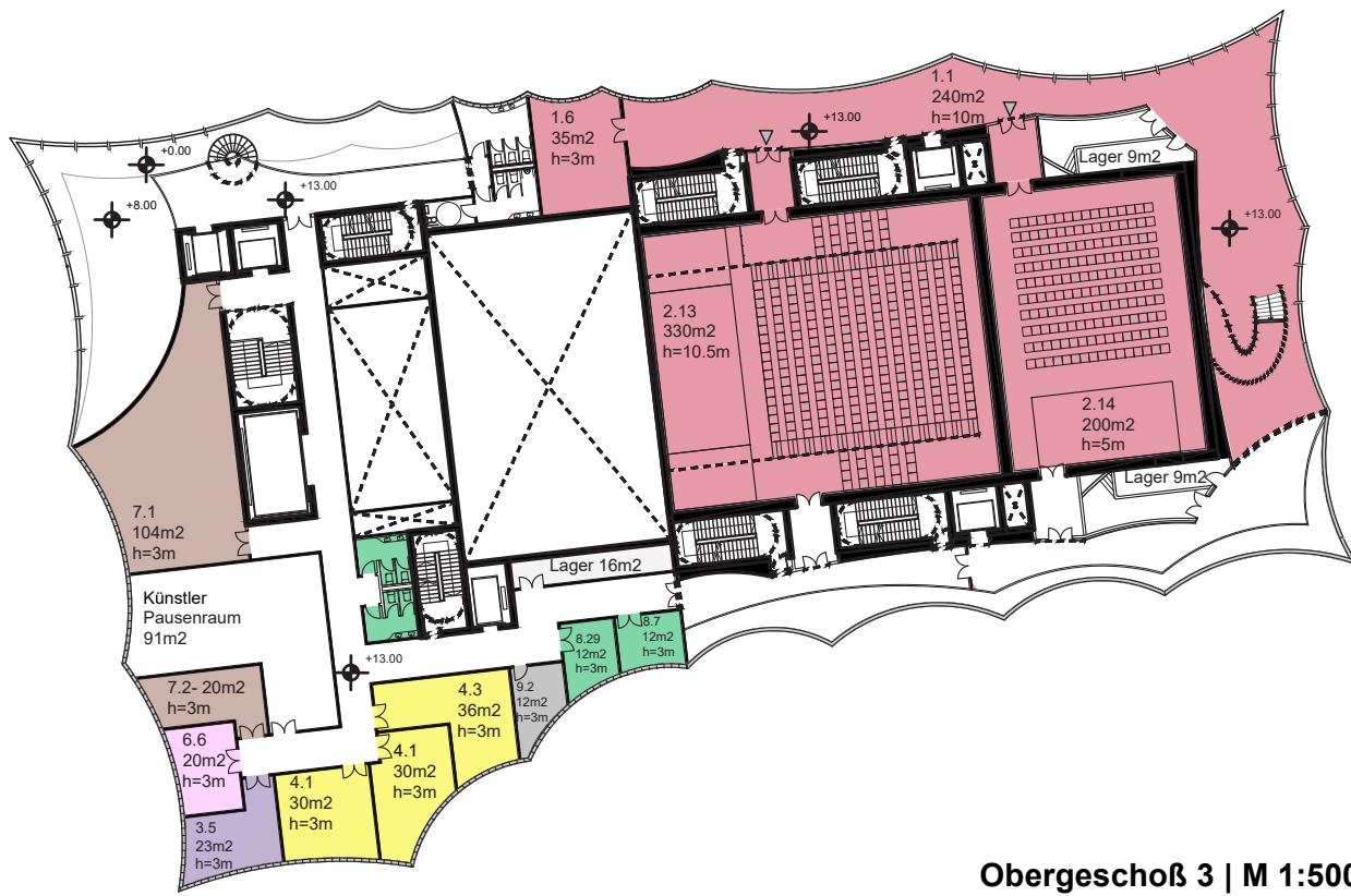
Obergeschoß 3 | M 1:500
