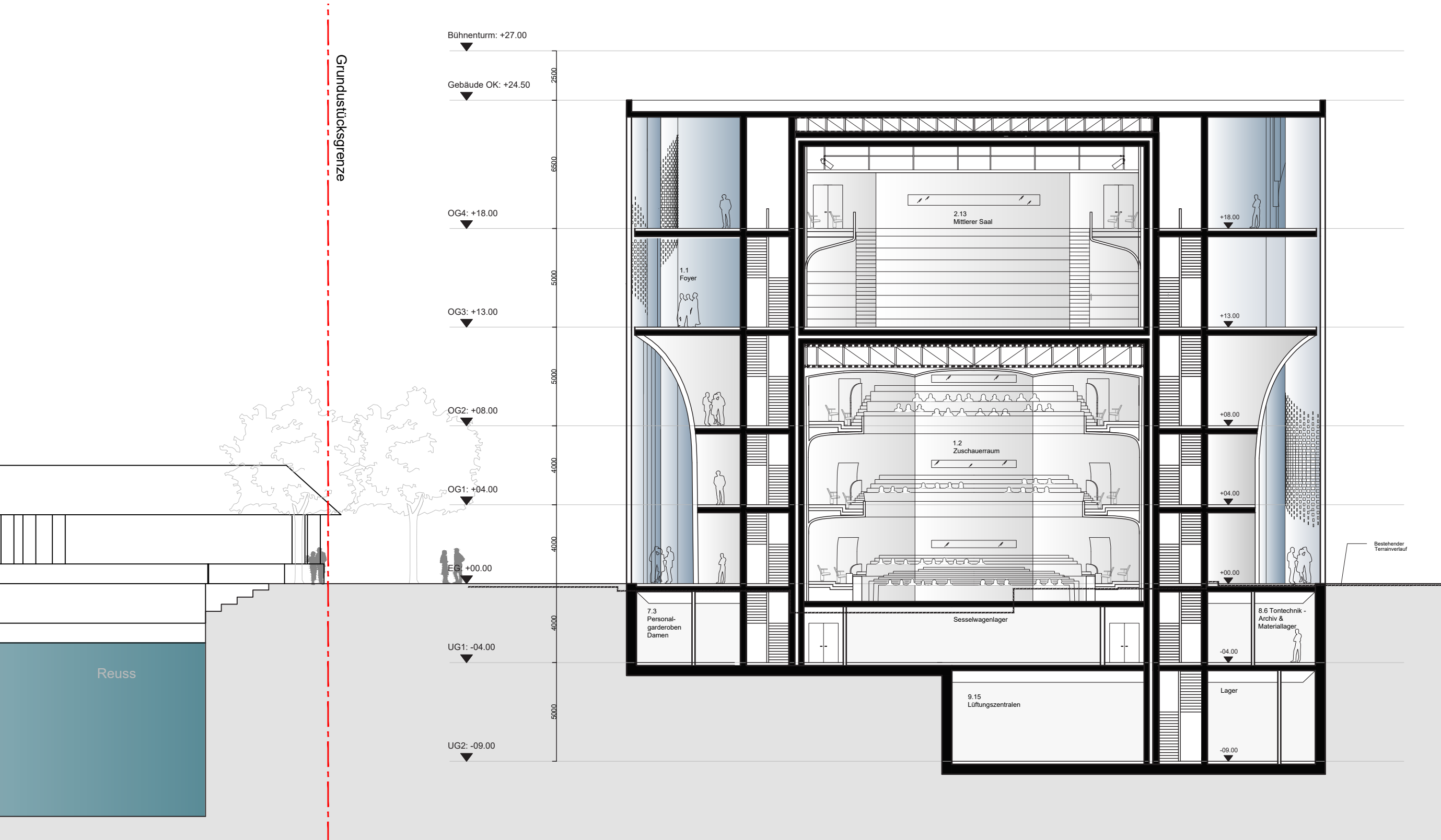
Querschnitt BB | M 1:200
