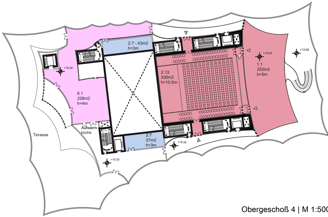
Obergeschoß 4 | M 1:500
