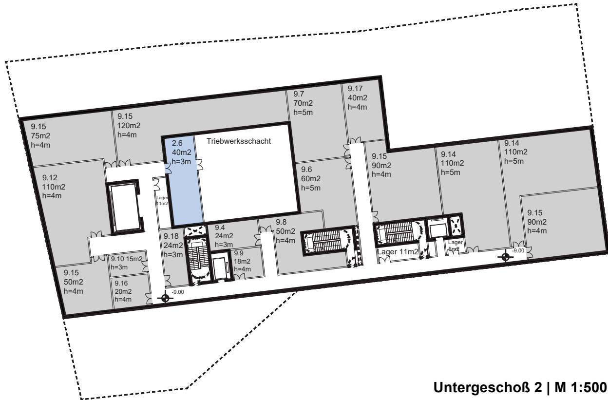
Untergeschoß 2 | M 1:500
