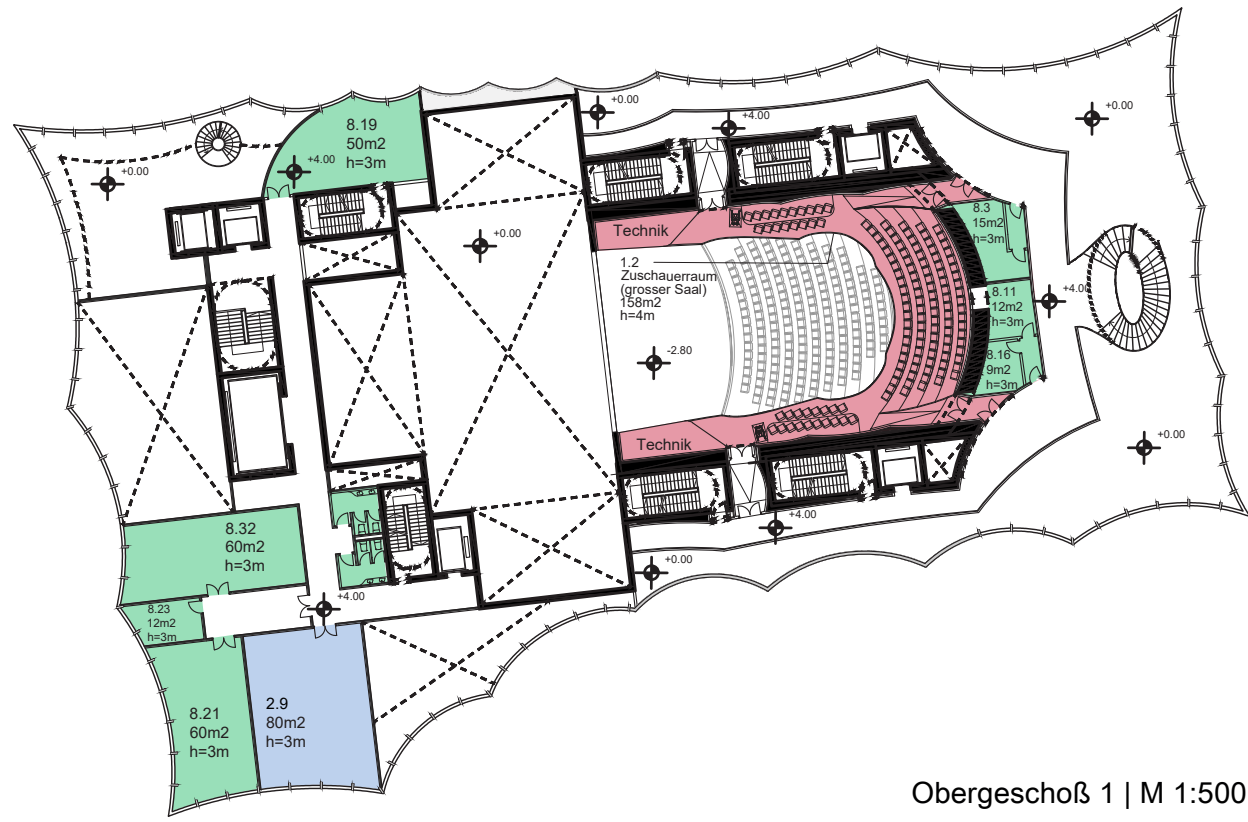
Obergeschoß 1 | M 1:500
