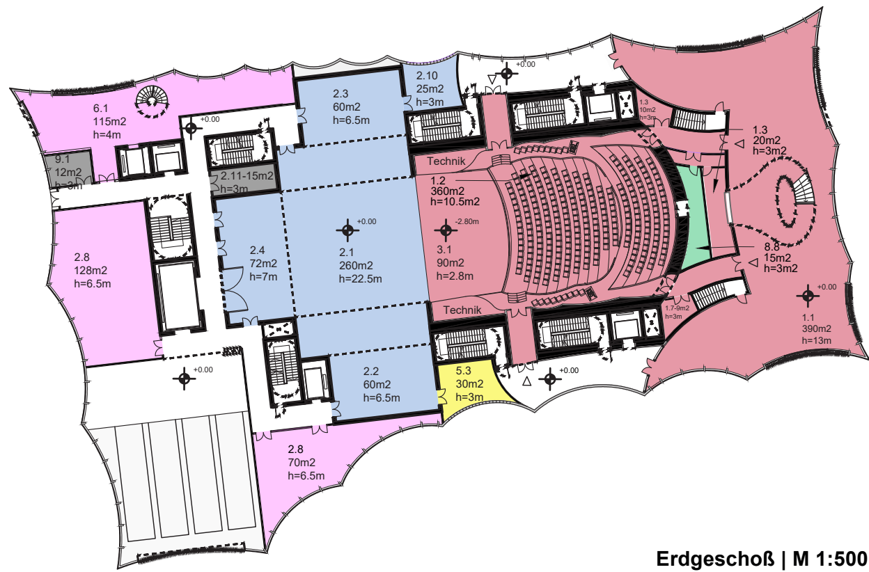
Erdgeschoß | M 1:500
