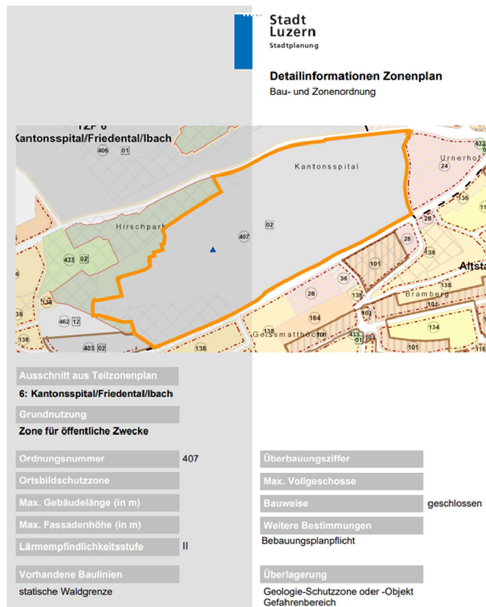
Abbildung 74: Auszug aus der Bau- und Zonenordnung für das LUKS-Areal
