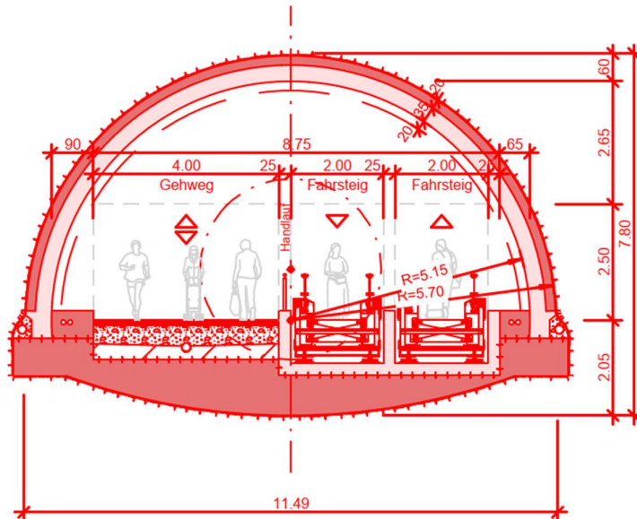
Abbildung 29: Normalprofil Stadtpassage hufeisenförmig, Variante Rollband
