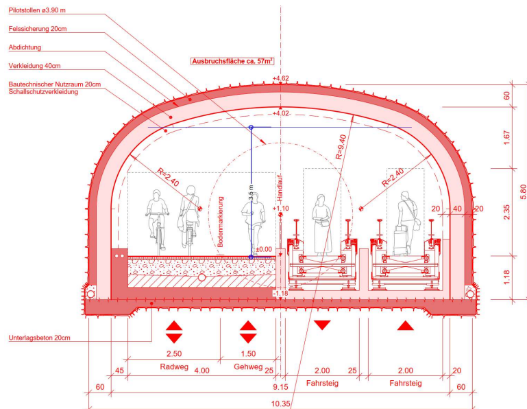
Abbildung 30: Normalprofil Stadtpassage gemäss IG Stadtpassage
