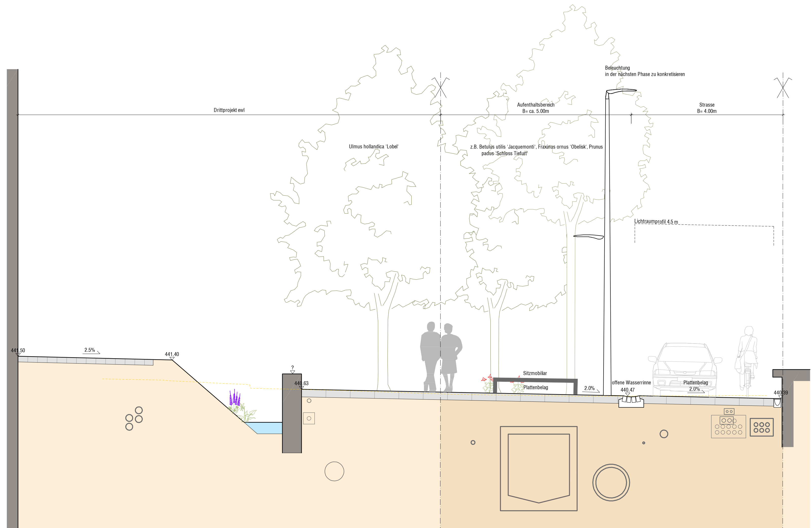
Querschnitt 18, 1:50
