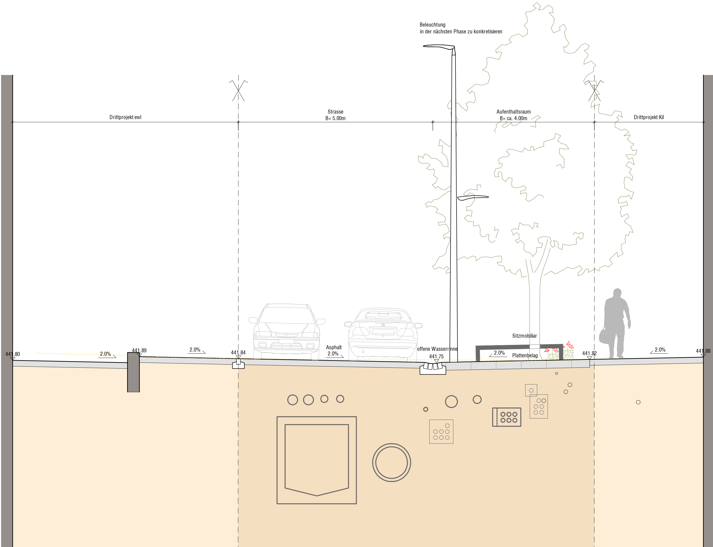
Querschnitt 4, 1:50
