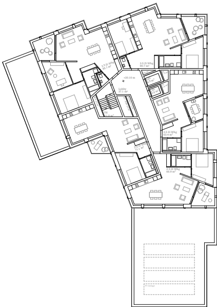
6. OBERGESCHOSS
