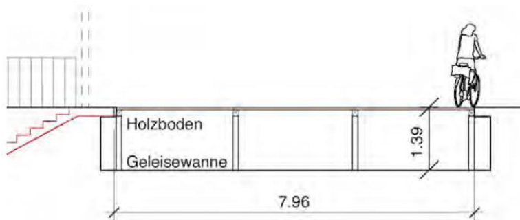
4.3.1 Abbildung Holzbohlenboden über den Gleisen
