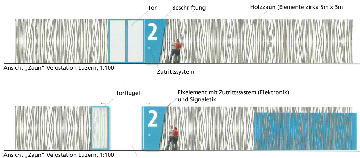
4.3.2 Abbildung Holzzaun
